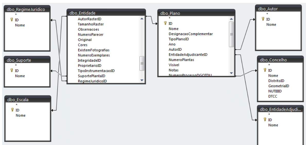
Fig. 2 - Base de dados AH-OTDU: Tabela dbo. Entidade (IGT - Peça desenhada) - Relações
