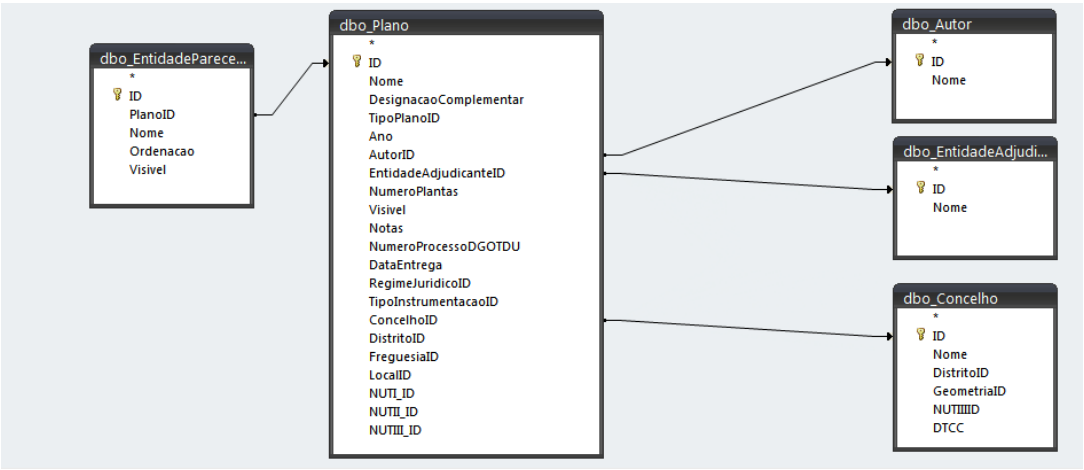
Fig. 4 - Base de dados AH-OTDU: Tabela dbo. EntidadeParecer (IGT - Pareceres CSOPT) - Relações
