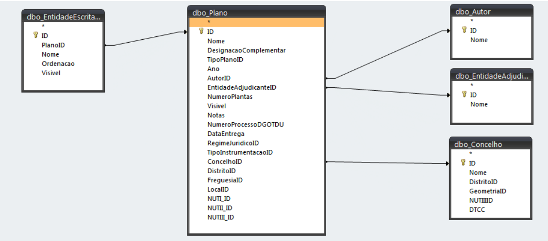
Fig. 3 - Base de dados AH-OTDU: Tabela dbo. EntidadeEscrita (IGT - Peça escrita) - Relações
