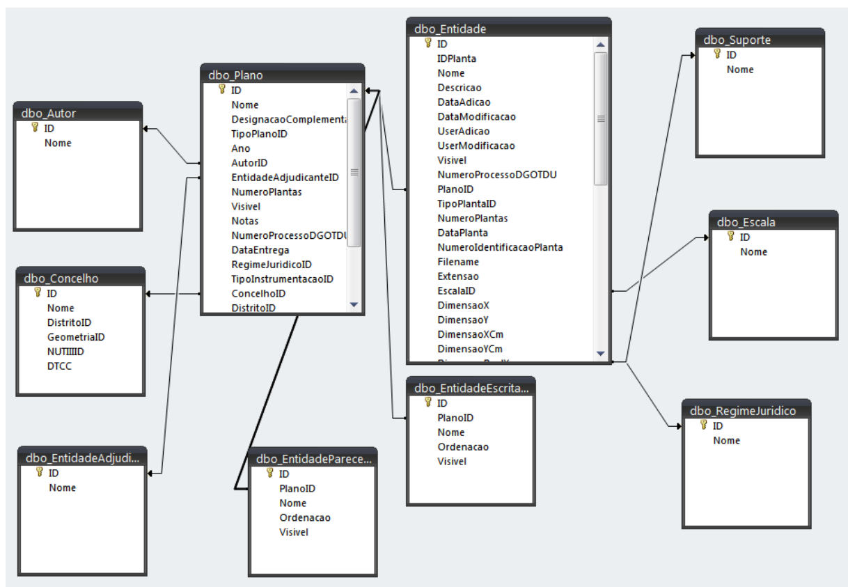
Fig. 1 - Base de dados AH-OTDU: Tabela dbo. Plano - Relações
