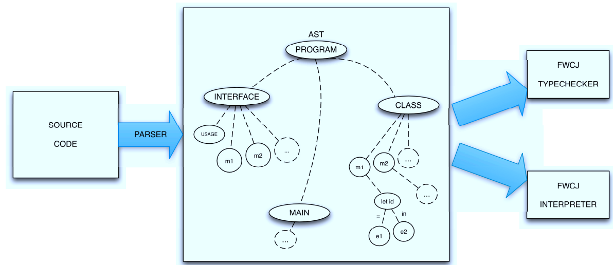
Figura 3.10: Fluxo geral de um programa
