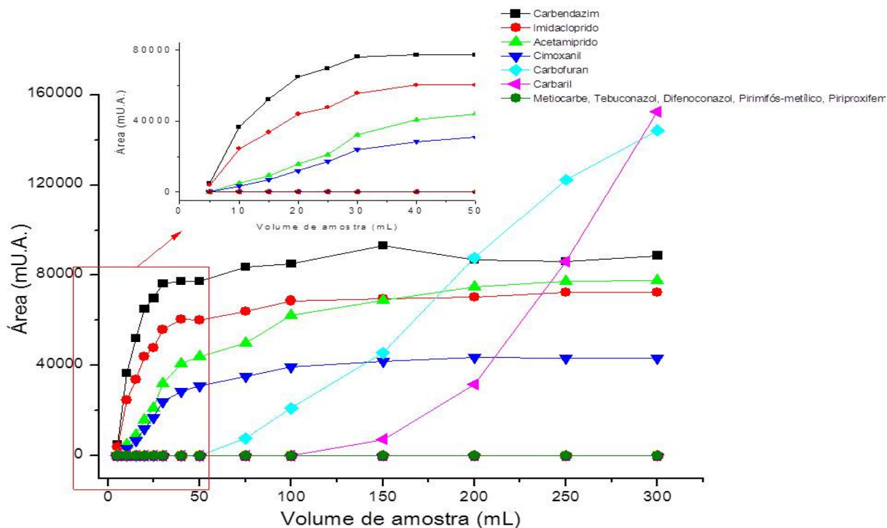
Figura 29: Curvas de breakthrough do cartucho de SiZrPMOS. Em destaque a região de volume de amostra de 0 a 50 mL.
