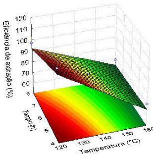
Metiocarbe - SiZrPMOS
