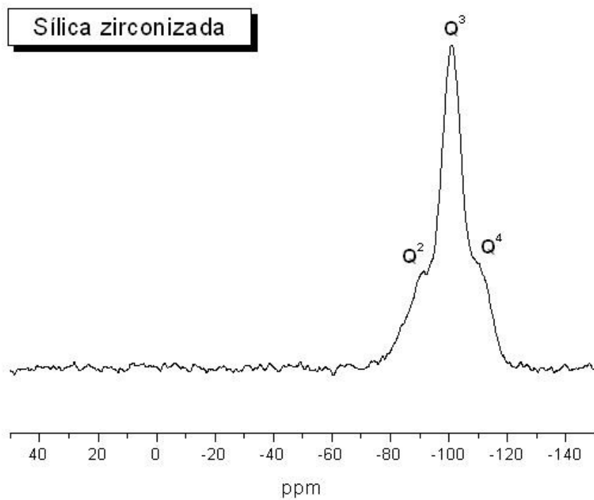
Figura 13: Espectros de RMN de ^{29}\text{Si} dos suportes de sílica não modificado e zirconizado.
