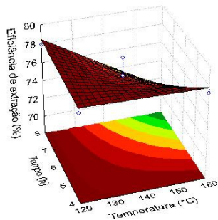
Pirimifós-metílico - SiZrPMOS
