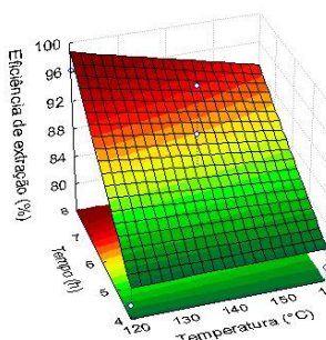
Pirimifós-metílico - SiPMOS
