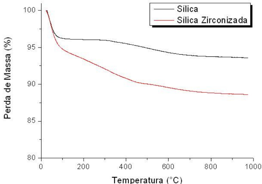
Figura 12: Curvas termogravimétricas dos suportes de sílica não modificado e zirconizado.
