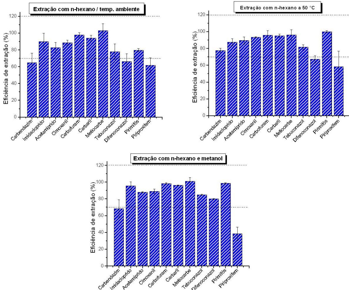
Figura 23: Eficiências de extração obtidas para os agrotóxicos em SiZrPMOS submetido a diferentes condições de extração do excesso de PMOS. As linhas tracejadas delimitam o intervalo aceitável, de 70 a 120% de eficiência de extração.
