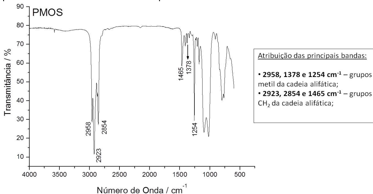
Figura 16: Espectro de absorção no infravermelho do PMOS. Em destaque a atribuição das principais bandas 52 .
