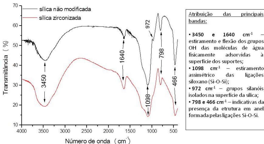
Figura 11: Espectros de absorção na região do infravermelho das amostras dos suportes de sílica não modificada e zirconizada. Em destaque a atribuição das principais bandas 52 .
