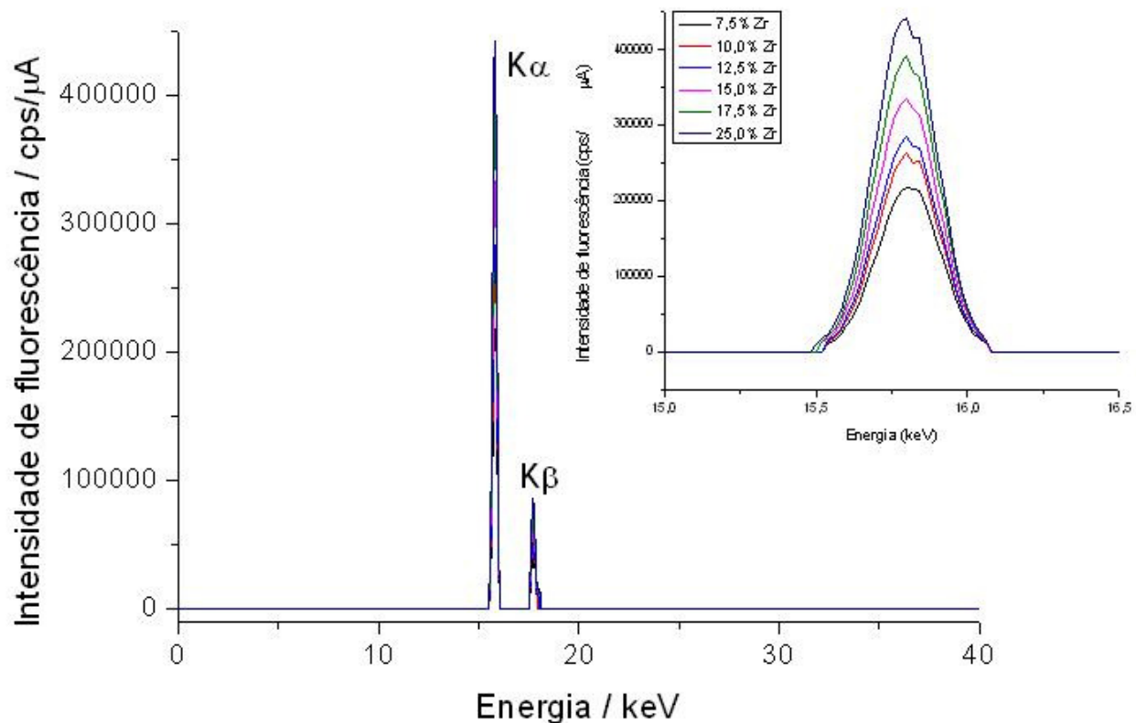
Figura 14: Espectros de fluorescência dos padrões de \text{SiO}_2/\text{ZrO}_2 utilizados para construção da curva analítica. Em destaque os picos K\alpha dos padrões com diferentes porcentagens em massa de zircônio.
