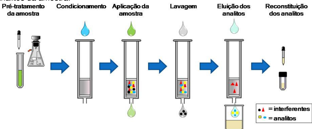
Figura 3: Etapas do procedimento de EFS no modo de concentração dos analitos.
