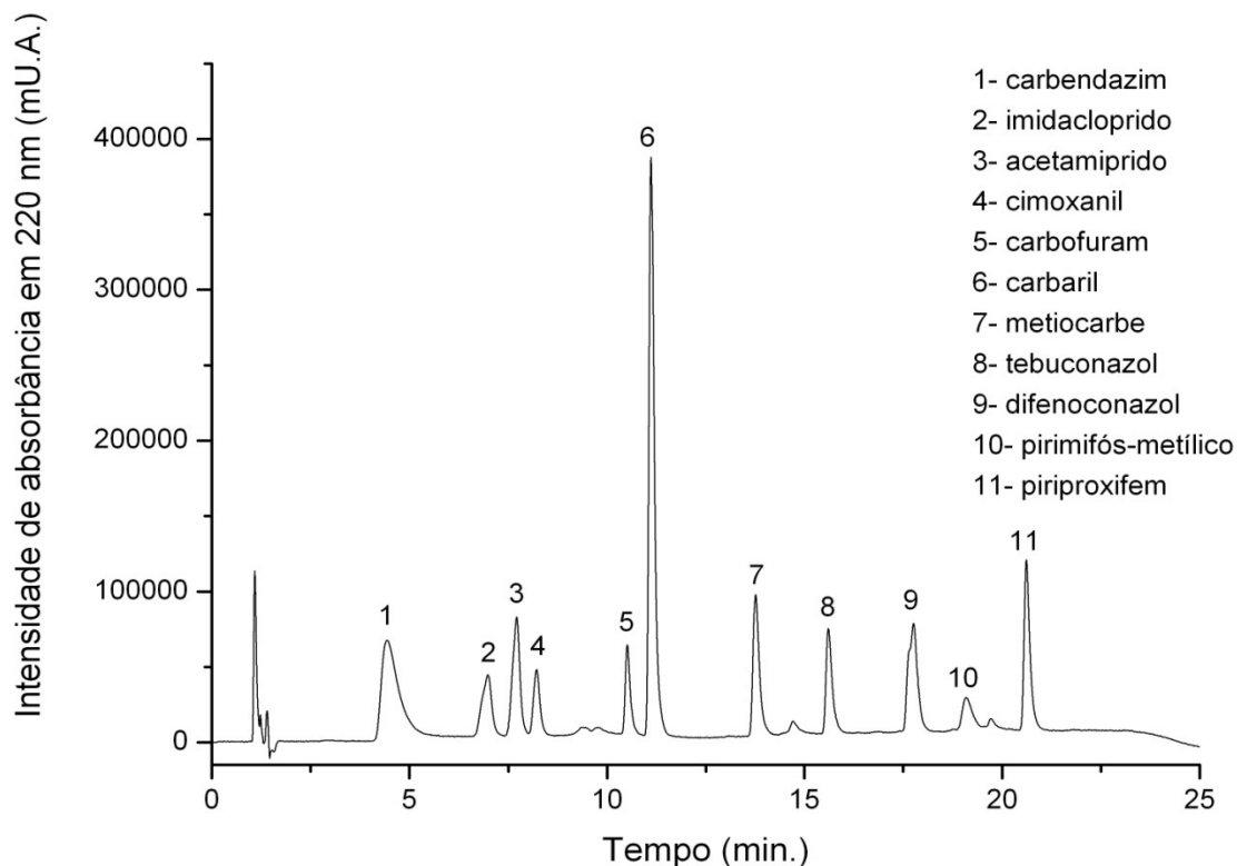
Figura 10: Cromatograma obtido em 220 nm na separação dos agrotóxicos estudados. Condições cromatográficas: volume de injeção de 17 \mu\text{L} ; coluna cromatográfica: NovaPak C18, Waters, 3,9x150 mm, partículas de 4 \mu\text{m} ; coluna de guarda: NovaPak C18, Waters, 3,9x20 mm, partículas de 4 \mu\text{m} ; fase móvel: água acidificada com ácido fosfórico a pH 2,5 (solvente A) e acetonitrila (solvente B); vazão de 1,0 \text{mL min}^{-1} ; programação do gradiente: 13 a 45% de B em 6 minutos, 45% de B por 2 minutos, 45 a 55% de B em 2 minutos, 55 a 95% de B em 10 minutos, 95% de B por 5 minutos, retorno às condições iniciais e estabilização por 10 minutos.
