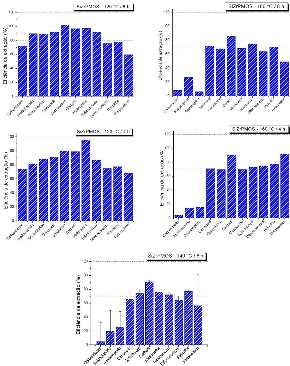
Figura 21: Eficiências de extração obtidas para os agrotóxicos extraídos em cartuchos de PMOS sobre sílica zirconizada em diferentes condições de imobilização. As linhas tracejadas delimitam o intervalo aceitável, de 70 a 120% de eficiência de extração.
