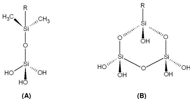
Figura 5: Representação de duas conformações dos sorventes quimicamente ligados: (A) estrutura monomérica, (B) estrutura polimérica.
