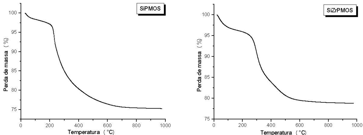
Figura 24: Curvas termogravimétricas dos sorventes preparados SiPMOS e SiZrPMOS.
