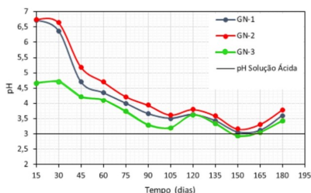
Figura 1. Comportamento médio do pH nas soluções residuais de hidrólise ácida de “granitos negros”, ao longo de sucessivos ciclos de experiências em bancada
