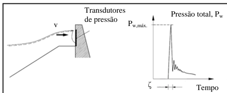
Figura 2.10: Forças de impulsos causadas pela rebenção da onda na superestrutura [adaptado de USACE, 2011].
