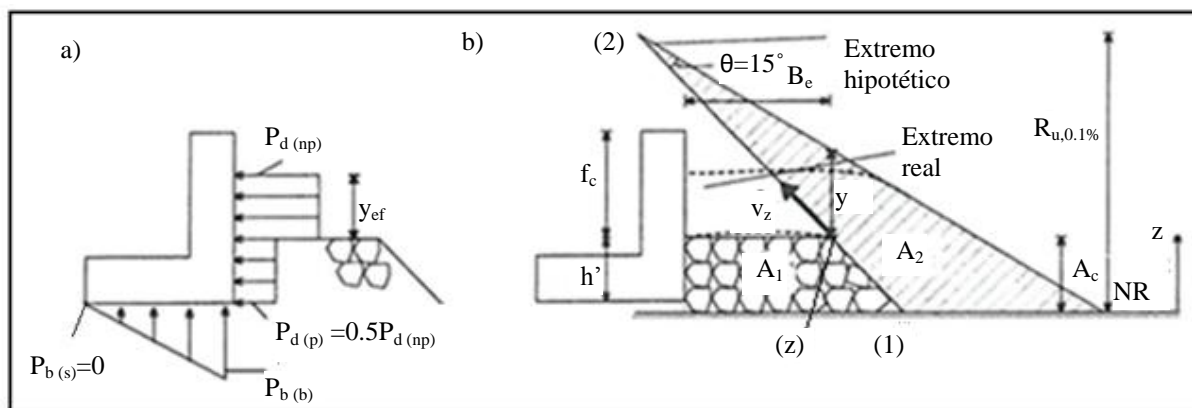
Figura 4.6: a) Distribuição de pressões na superestrutura proposta por Pedersen, 1996. b) Traçado da cunha de espraioamento e os parâmetros de cálculo [adaptado de Pedersen, 1996].
