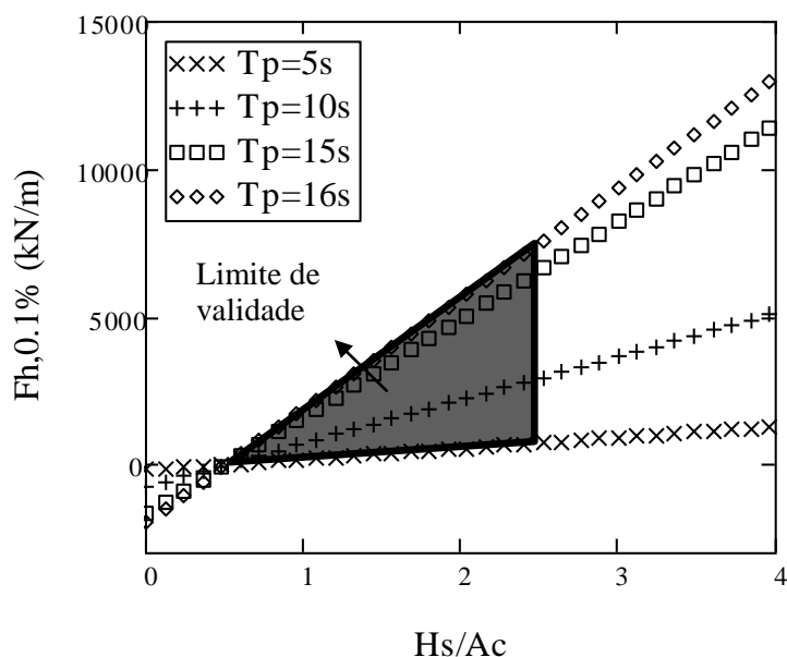
Figura 5.1: Variação de F_{h,0.1\%} com H_s/A_c , para diferentes valores de T_p .
