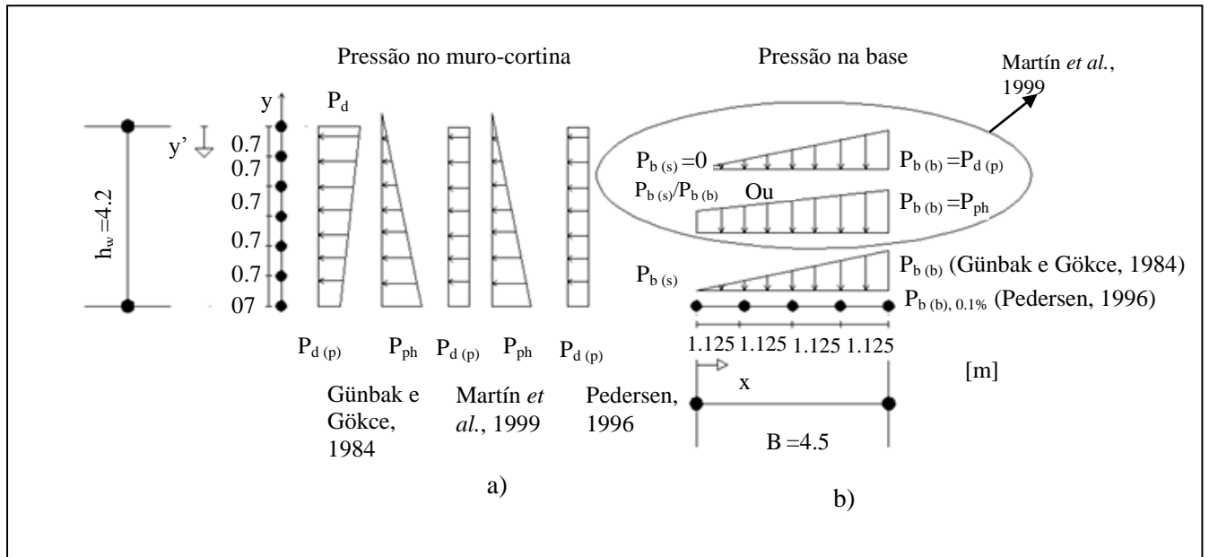
Figura 6.11: Diagrama de pressões para as 3 formulações em análise neste ponto: a) Pressão no muro-cortina. b) Pressão na base.
