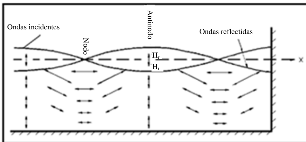
Figura 3.7: Representação esquemática de ondas incidentes e ondas refletidas num regime estacionário [adaptado de USACE, 2008].
