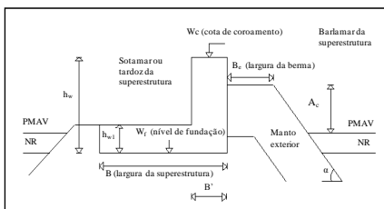
Figura 1: Características geométricas de uma superestrutura
