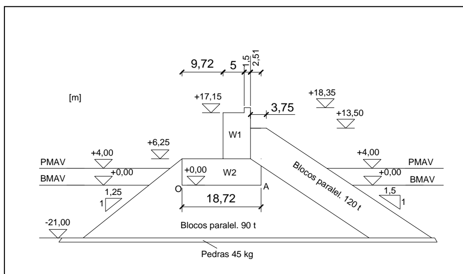
Figura 6.1: Secção transversal do quebra-mar de talude do Porto de Gijón [adaptado de Martín et al. , 1999a].
