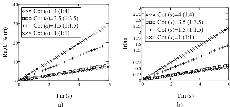
Figura 5.28: a) Variação de R_{u,0.1\%} com T_m para diferentes valores de cot(α). b) Variação de Ir_{0m} com T_m para diferentes valores de cot(α).
