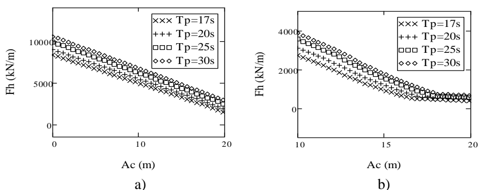
Figura 5.41: a) Variação de F_h com T_p para diferentes valores de A_c . b) Variação de F_h com T_p para diferentes valores de A_c dentro de limite de validade da fórmula.
