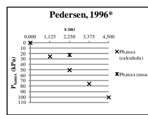
Figura 5: Pressões na base: formulação de Pedersen, 1996
