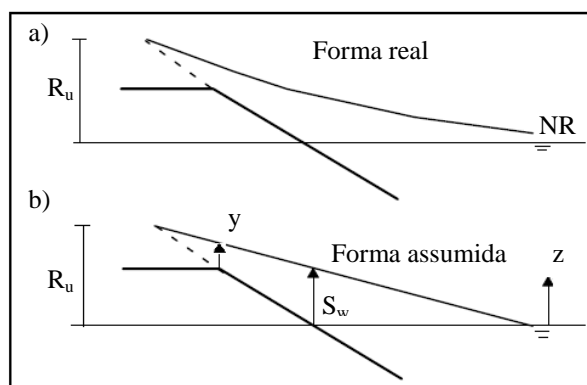
Figura 4.11: Perfil simplificado de espraiamento [adaptado de Martín et al. , 1999b].
