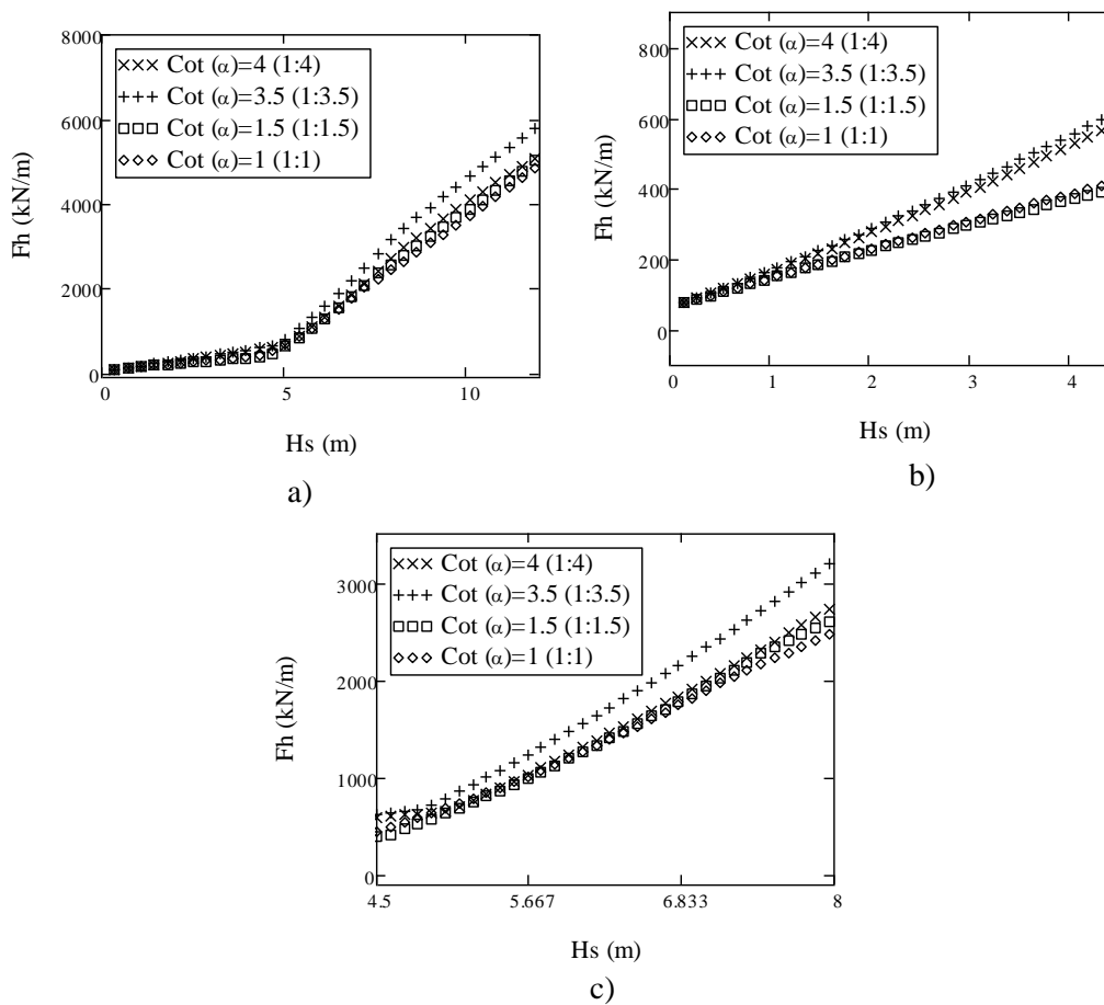
Figura 5.42: a) Variação de F_h (P_d + P_{ph}) com H_s para diferentes valores de \cot(\alpha) . b) Variação de F_h (P_{ph}) com H_s para diferentes valores de \cot(\alpha) dentro do limite de validade. c) Variação de F_h (P_d) com H_s para diferentes valores de \cot(\alpha) dentro do limite de validade.
