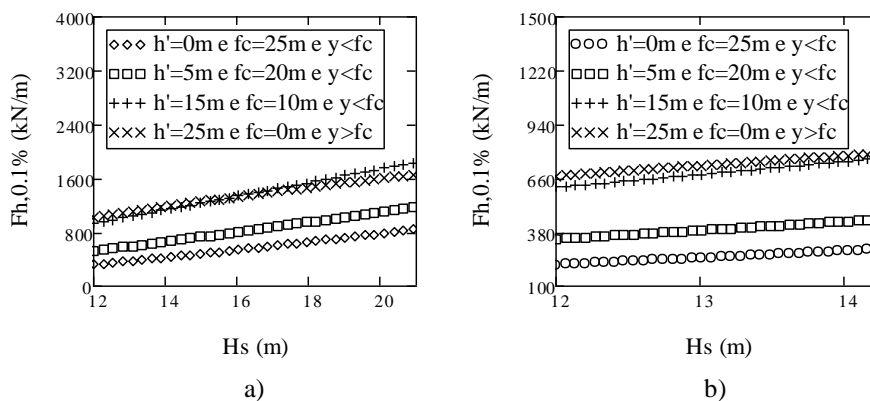
Figura 5.33: a) Variação de F_{h,0.1\%} com H_s para diferentes valores de h' e f_c . b) Variação de F_{h,0.1\%} com H_s para diferentes valores de h' e f_c dentro dos limites de validade.
