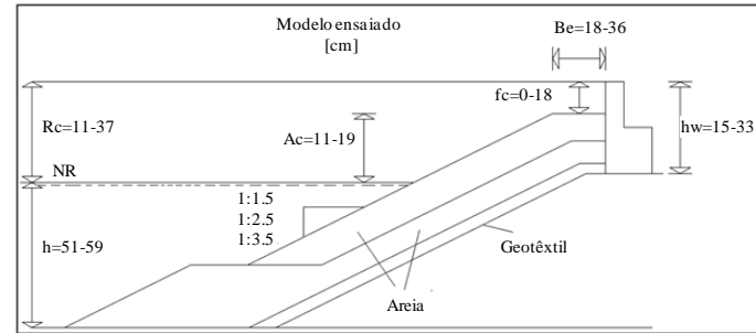
Figura 9: Seção transversal da superestrutura ensaiada por Pedersen [Pedersen, 1996]
