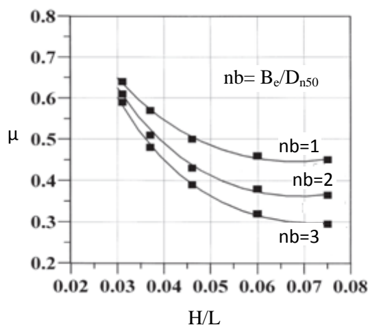
Figura 4.13: Valores de \mu proposto por Martín et al. , 1999 [Martín et al. , 1999a].
