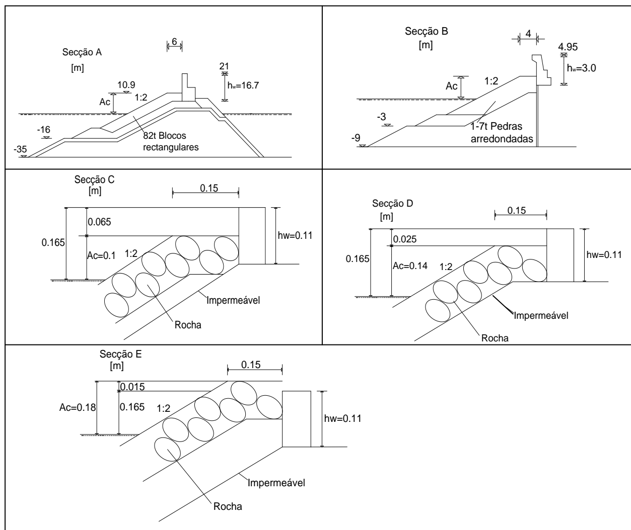
Figura 4.3: Secção transversal da superestrutura ensaiada por estes autores [adaptado de USACE, 2011].
