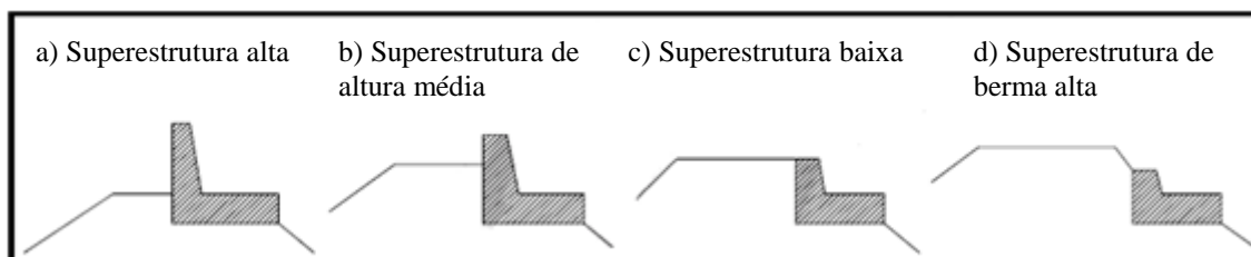
Figura 2.3: Configurações típicas de uma superestrutura [adaptado de USACE, 2011].
