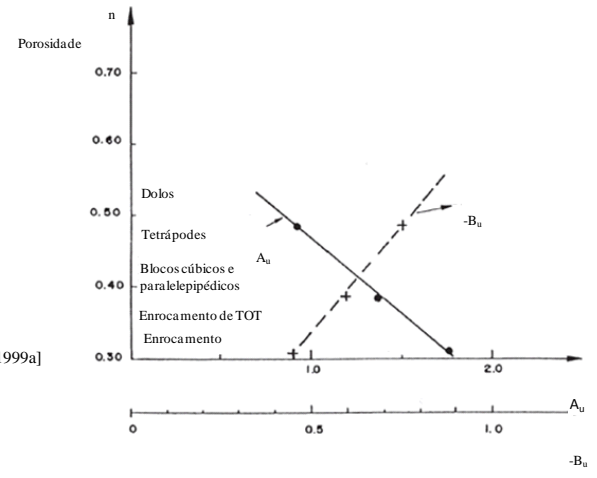
Figura 12: Coeficientes empíricos A_u e B_u para cálculo de espraio em função da porosidade do material que constitui o manto principal exterior [Martín et al. , 1999a]
