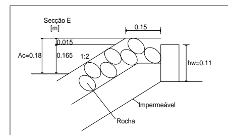
Figura 8: Secções transversais de superestruturas ensaiadas por Jensen, 1984, Bradbury et al. , 1988 [USACE, 2011].
