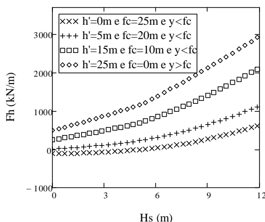
Figura 5.8: Variação de F_h com H_s para diferentes valores de h' e f_c .
