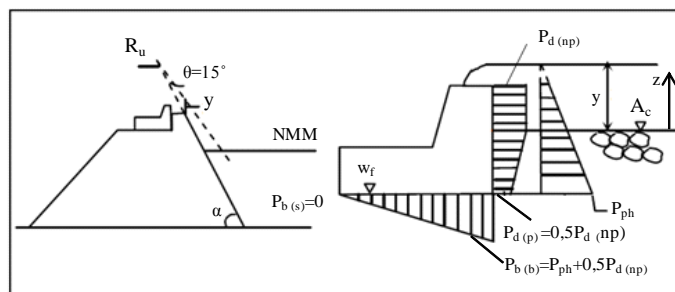
Figura 11: a) Traçado da cunha de espraioamento e os parâmetros de cálculo b) Distribuição de pressão na base e na face frontal da superestrutura [Martínez, 2001a]
