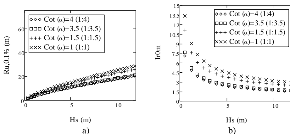
Figura 5.19: a) Variação de R_{u,0.1\%} com H_s para diferentes valores de \cot(\alpha) .
