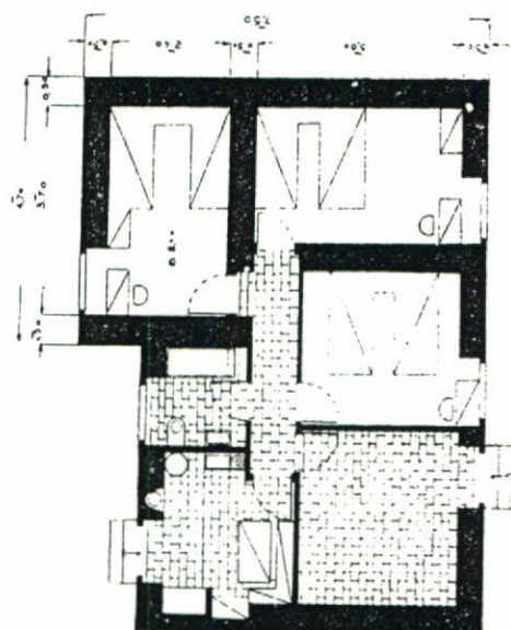
Portimão - Bairro Operário - Alçado e plantas das casas do tipo n.º 1, destinadas a casais sem filhos. Ampliações previstas para 2 e 3 quartos
