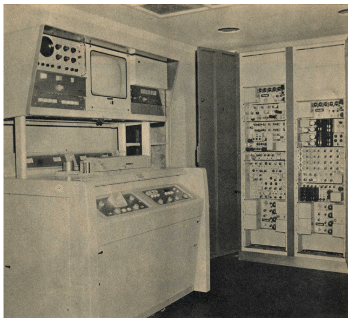
Ilustração 15. Videotape AMPEX VR-1000 ( TV Semanário da Radiotelevisão Portuguesa , 19 de março de 1964)
