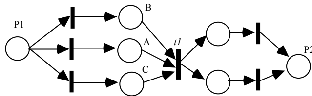
Figura 2.15- Transformação de RdP Generalizada da Figura 2.14 em Normal
