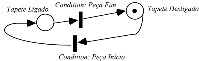
Figura 4.19 - RdP para Descrever Funcionamento de um Tapete - PTN
