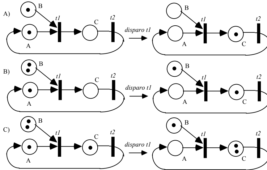
Figura 2.10 - Exemplos de Disparo de RdPs
