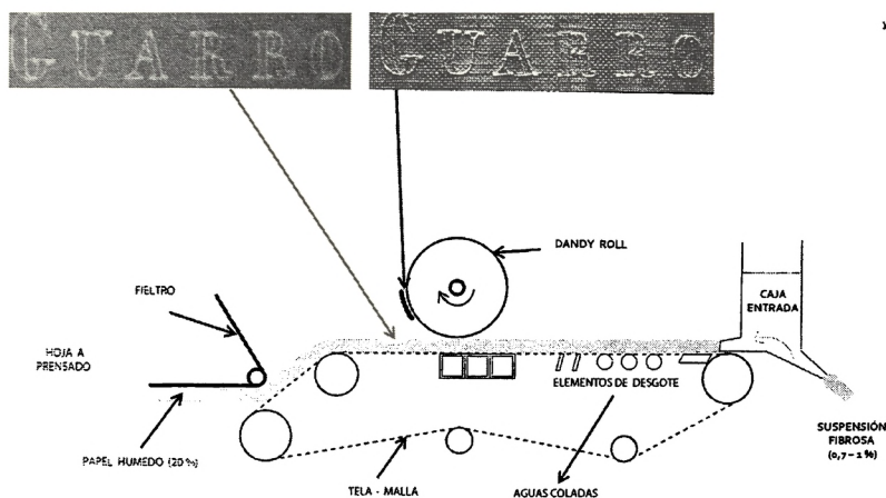
Imagen 3. Formación de la hoja de papel en mesa plana Fourdrinier.
