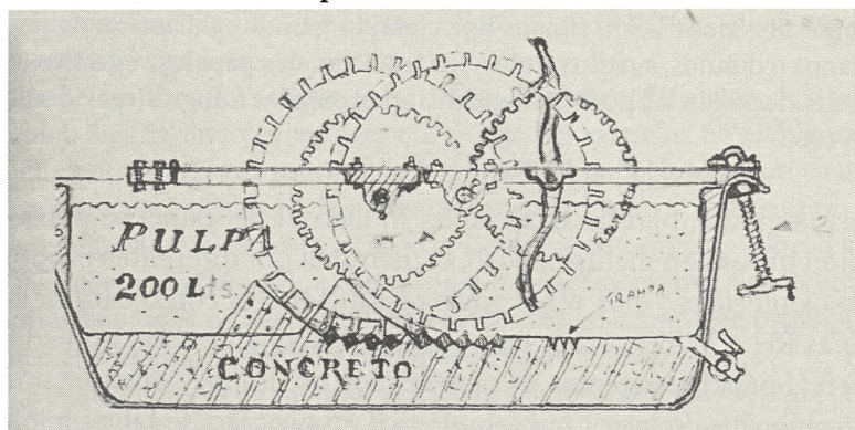
Imagen 2. Plano de pila holandesa diseñado y dibujado por Per Anderson.
