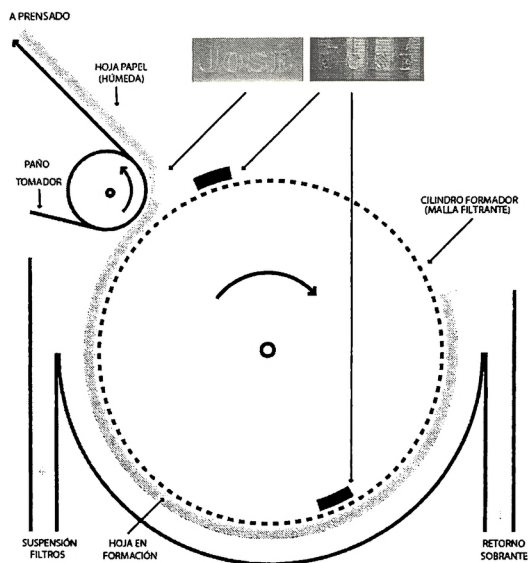
Imagen 4. Formación de la hoja de papel en máquina de forma redonda
