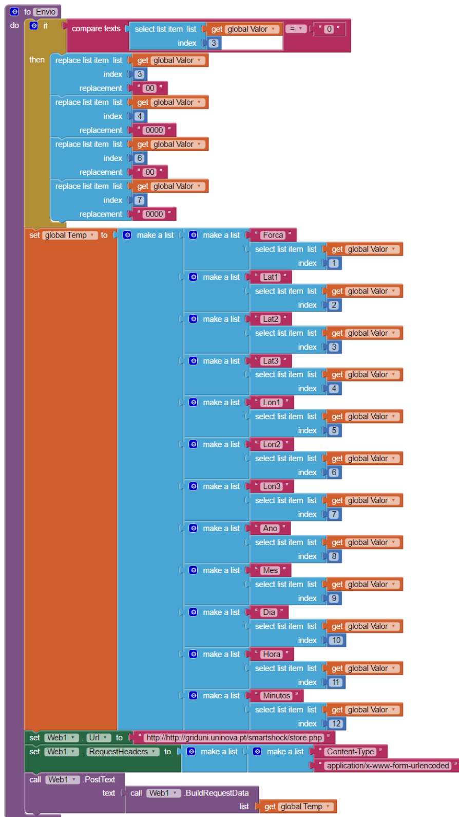
Figura B.6: Transformação de variáveis para envio para a base de dados
