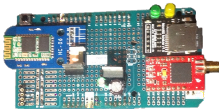
Figura 4.11: Montagem real do sistema
