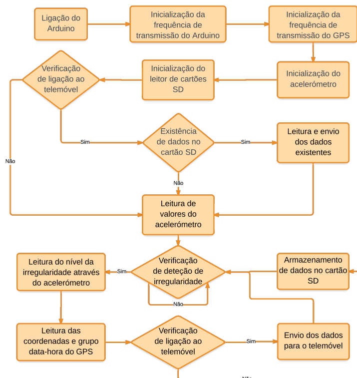
Figura 4.2: Fluxograma referente ao código Arduino
