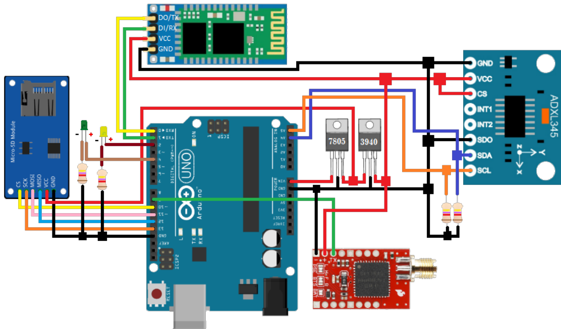
Figura 4.10: Esquemático do sistema
