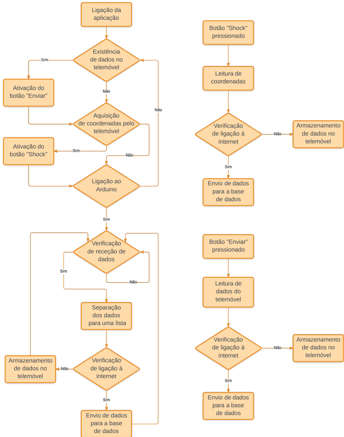
Figura 4.6: Fluxograma referente ao código Android
