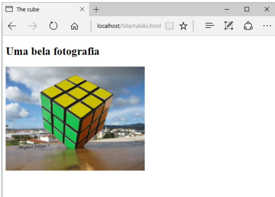
Figura 3.8: Exemplo de código HTML e o resultado num browser
