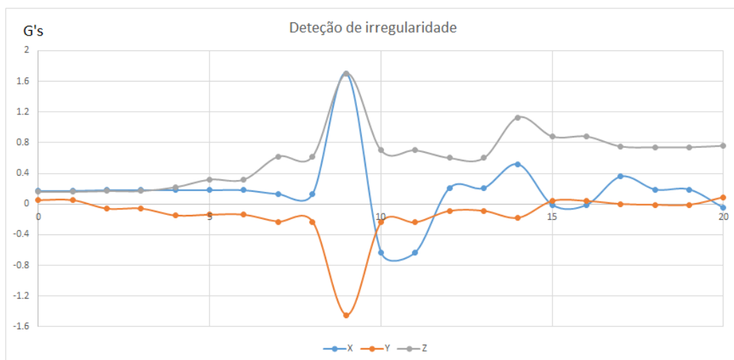
Figura 4.3: Gráfico de uma irregularidade detetada
