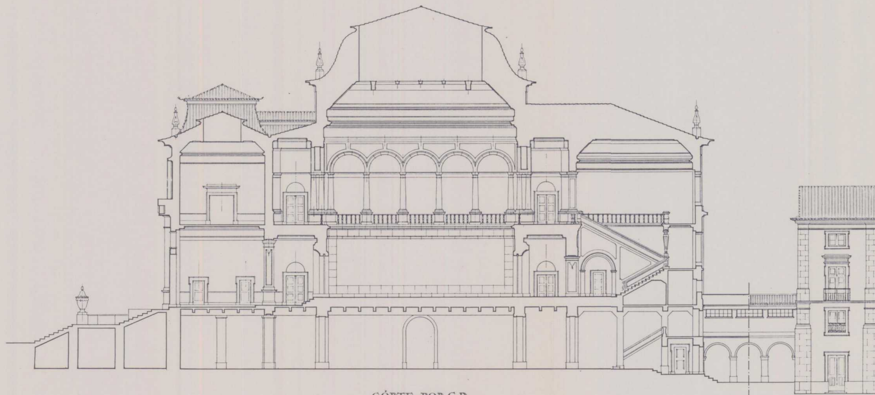
CÔRTE POR C D
