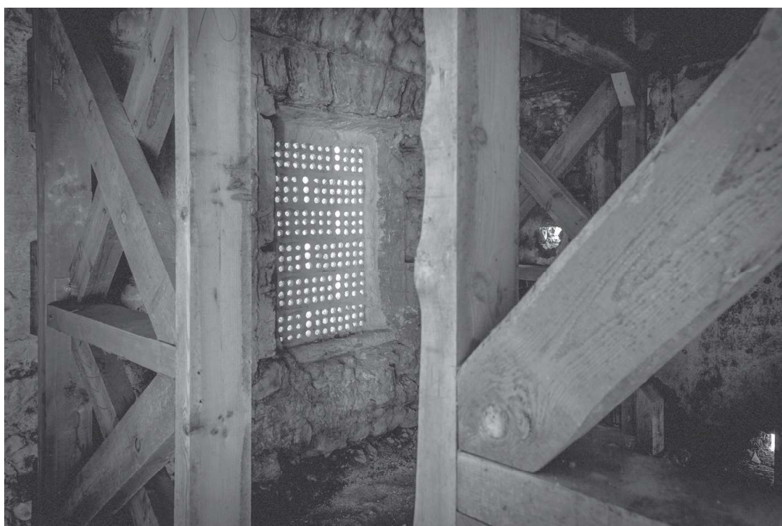
Fig. 7. Convento dos Capuchos, Setúbal: tijolo furado enquanto filtro de luz (2016). Fonte: José Manuel.
