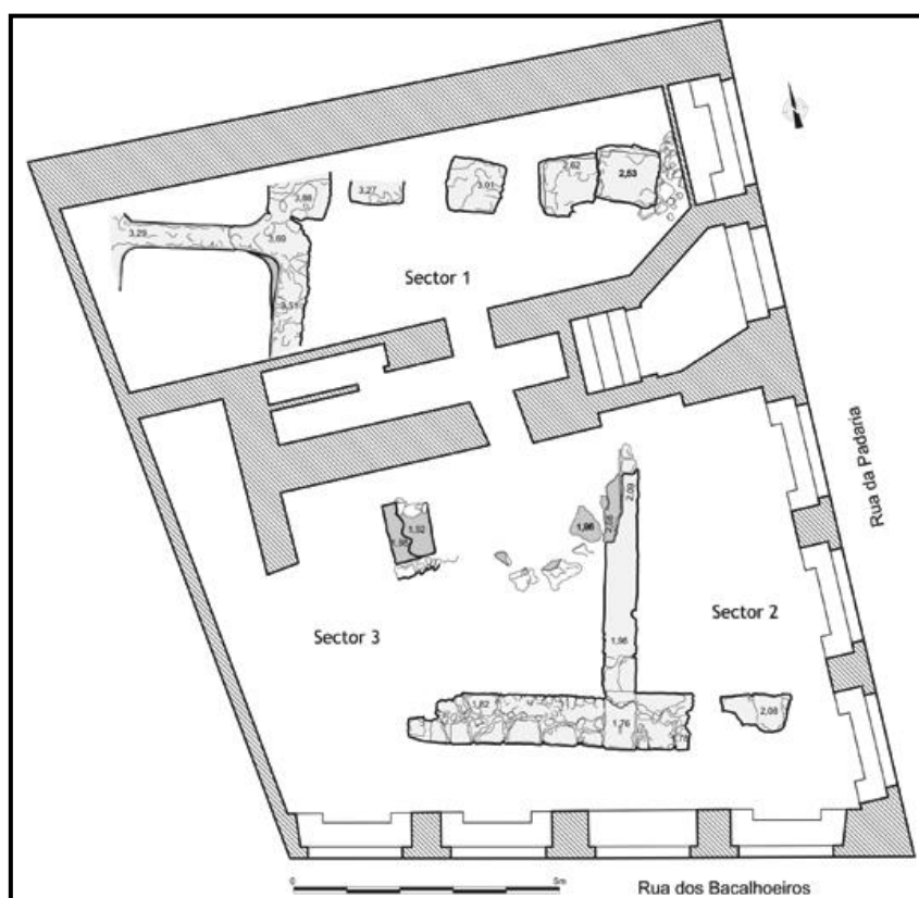
Figura 60- Planta de síntese das estruturas romanas exumadas na intervenção arqueológica da Rua dos Bacalhoeiros (segundo Vítor Filipe 1723 ).
