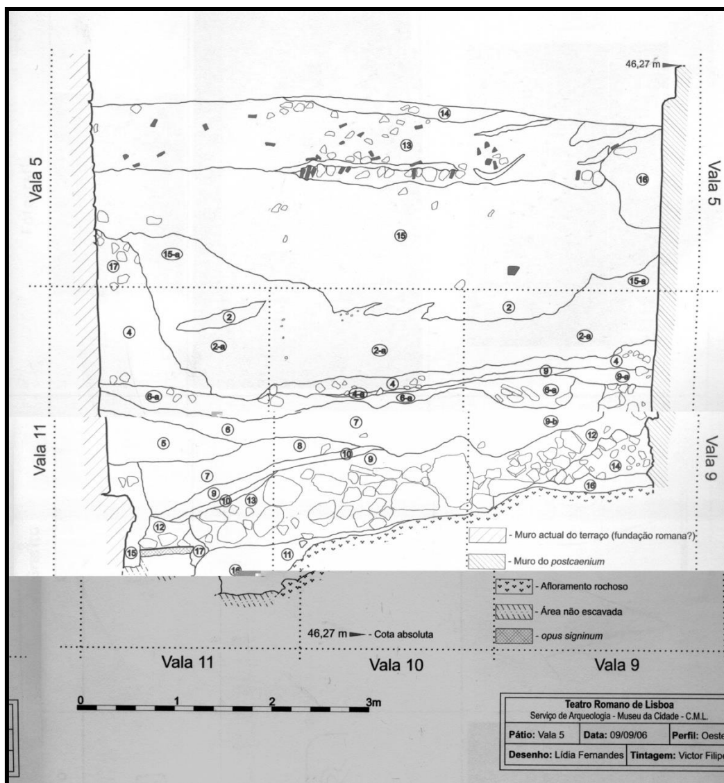
Figura 35- Perfil exterior e perpendicular ao postscenium (seg. Vítor Filipe 1444 ).
