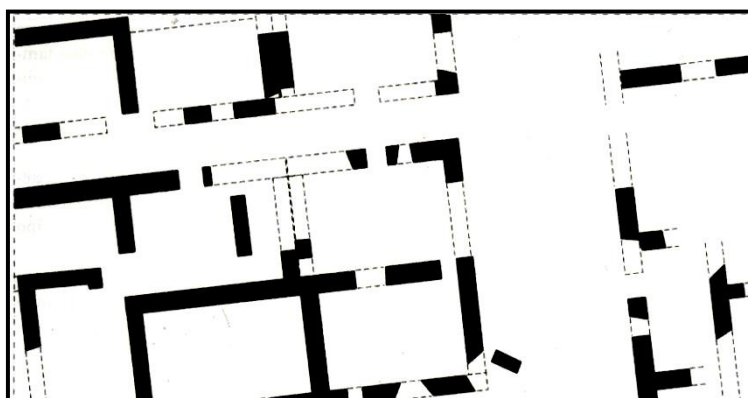
Figura 168- O urbanismo romano do período tardo-republicano (fase 1) patenteado pela escavação dos “Viveiros do Jardim”- 1999/2001 (segundo Catarina Viegas 2903 ).
