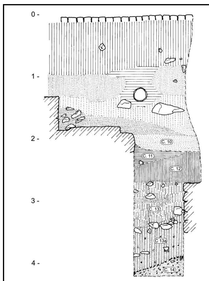
Figura 48- Perfil estratigráfico da zona do embasamento interno da muralha romana (segundo João Pimenta, Marco Calado e Manuela Leitão 1644 ).
