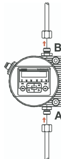
Figura 1-2 – representação esquemática do modo de instalação do TCM
