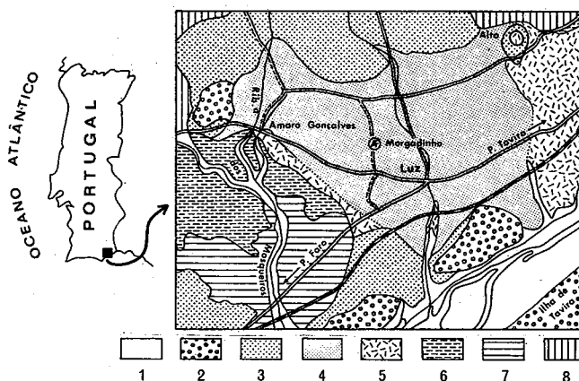
Fig. 1 — Emplacement du gisement de Morgadinho (AF), selon la carte géologique 1:50 000 de Tavira (MANUPPELLA et al. , 1984). 1 — alluvions; 2 — sables et graviers quaternaires; 3 — silts et sables fins quaternaires; 4 — dépôts de Morgadinho, Villanyien à Biharien; 5 — Formation de Cacela, Tortonien supérieur et Messinien; 6 — Crétacé inférieur; 7 — Portlandien B; 8 — Kimmeridgien-Portlandien A
