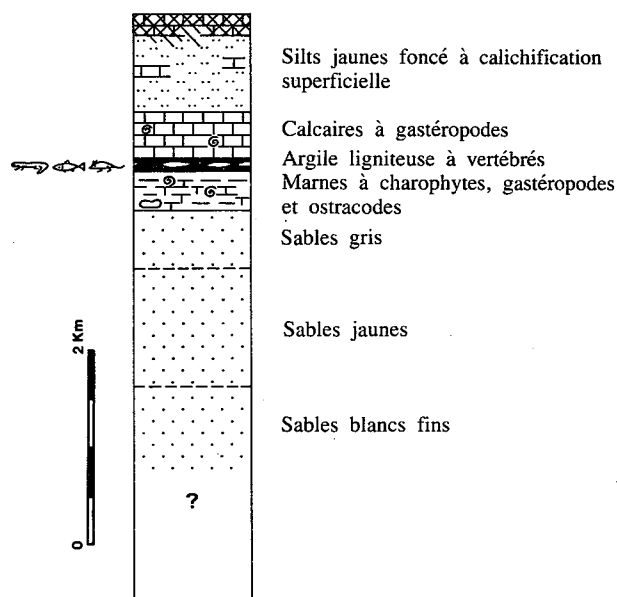
Fig. 2 — Coupe géologique schématique du puits de Morgadinho
